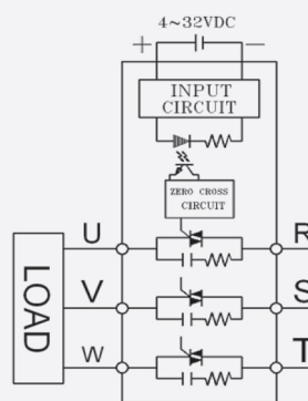
TSR-25DA-□ / TSR-40DA-□
