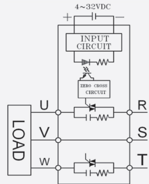
TSR-50DA-□ / TSR-75DA-□
